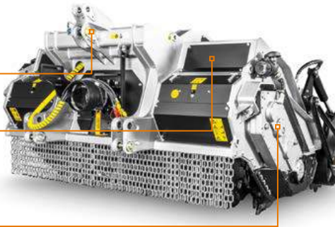
Placas de desgaste internas em Hardox® aparafusadas Garantem resistência superior ao desgaste e a danos.
