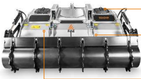
Dispositivo de autoalinhamento estilo W entre o cardan e a caixa de engrenagens da tomada de força (PTO) Permite que o triturador trabalhe em diversos ângulos sem danificar o cardan.
