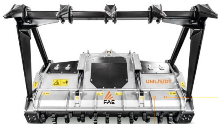
Láminas internas con revestimiento anti desgaste FCP
